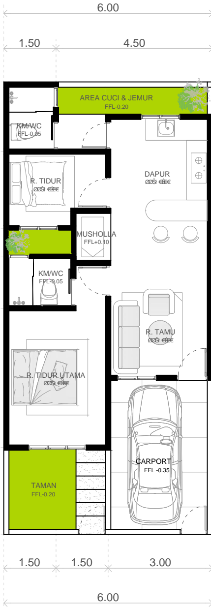
DENAH Type 75 Skala : 1 :100
